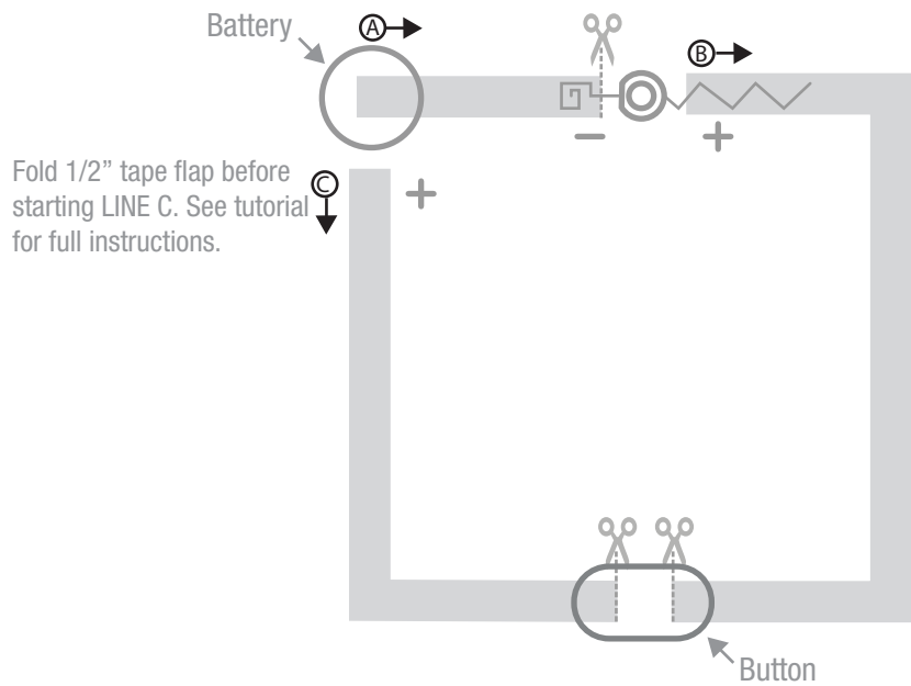
Pixel Heart Circuit Template
